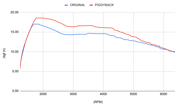
TORQUE DE RODA (kgf.m)
