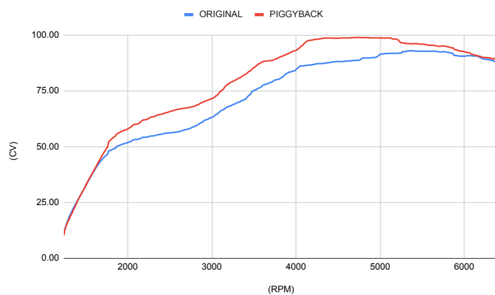
POTÊNCIA DE RODA (CV)
