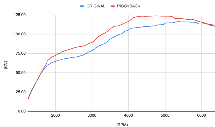
POTÊNCIA DE MOTOR (CV)
