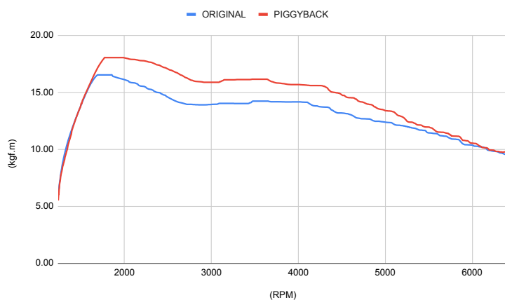
TORQUE DE MOTOR (kgf.m)
